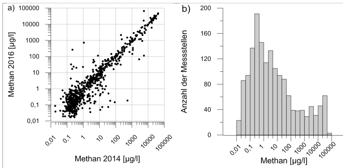
Abb. 8: a) Vergleich der Methankonzentrationen von ca. 700 Grundwassermessstellen, b) Häufigkeitsverteilungen der Methankonzentrationen aller beprobten Grundwassermessstellen (n = 1605). Pro Messstelle wird nur der aktuellste Messwert herangezogen. Abbildungen a) und b) sind modifiziert nach SCHLOEMER et al. (2018).
