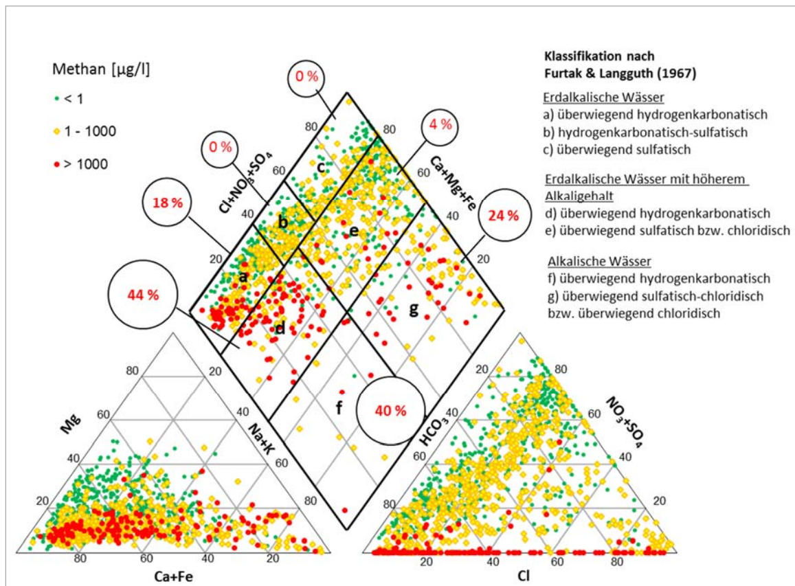
Abb. 10: Hydrochemische Auswertung der Proben im Piper-Diagramm. Die Proben werden nach FURTA & LANGGUTH (1967) in Grundwassertypen klassifiziert. Der Anteil der Proben mit Methankonzentrationen >1000 \mu\text{g/l} an den Wassertypen ist in den Kreisen angegeben.
