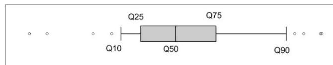
Abb. 11: Darstellung der Konzentrationen mit Hilfe eines Boxplots. Die Box entspricht hierbei dem Konzentrationsbereich, in dem 50 % der Werte liegen. Der Beginn der Box stellt das untere Quartil (Q25), der Strich innerhalb der Box den Median (Q50) und das Ende der Box das obere Quartil (Q75) dar. Die Whisker entsprechen dem 10. und 90. Perzentil (Q10 und Q90). Die Punkte außerhalb der Whisker geben die unteren bzw. oberen 10 % der Verteilung wieder (WALSER 2011).
