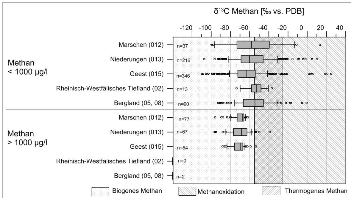
Abb. 23: Verteilung der \delta^{13}\text{C} -Werte des Methans in den Marschen, Niederungen, Geestgebieten und im Bergland, untergliedert in die Proben mit Methankonzentrationen größer und kleiner 1000 \mu\text{g/l} .
