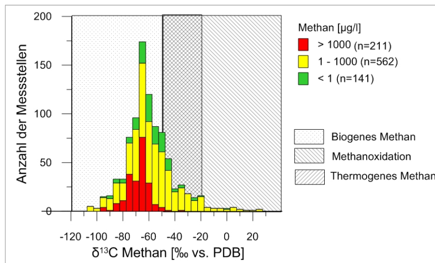
Abb. 9: \delta^{13}\text{C} -Werte von Methan (n = 914). Pro Messstelle wird nur der aktuellste Messwert herangezogen. Abbildung modifiziert nach SCHLOEMER et al. (2018).
