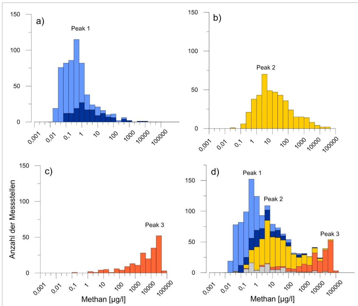
Abb. 13: Häufigkeitsverteilungen der Methankonzentration, untergliedert in die vier Reduktionsgrade a) \text{O}_2\uparrow ( n = 446 ) und \text{O}_2\downarrow , \text{NO}_3\uparrow ( n = 146 ), b) \text{O}_2\downarrow , \text{NO}_3\downarrow und \text{SO}_4\uparrow ( n = 438 ) sowie c) \text{O}_2\downarrow , \text{NO}_3\downarrow und \text{SO}_4\downarrow ( n = 195 ). In d) ist das Histogramm der Gesamtkonzentration unterteilt in die vier Reduktionsgrade. Proben, welche keinem der vier Reduktionsgrade zugeordnet werden konnten, wurden in Grau dargestellt ( n = 81 ).
