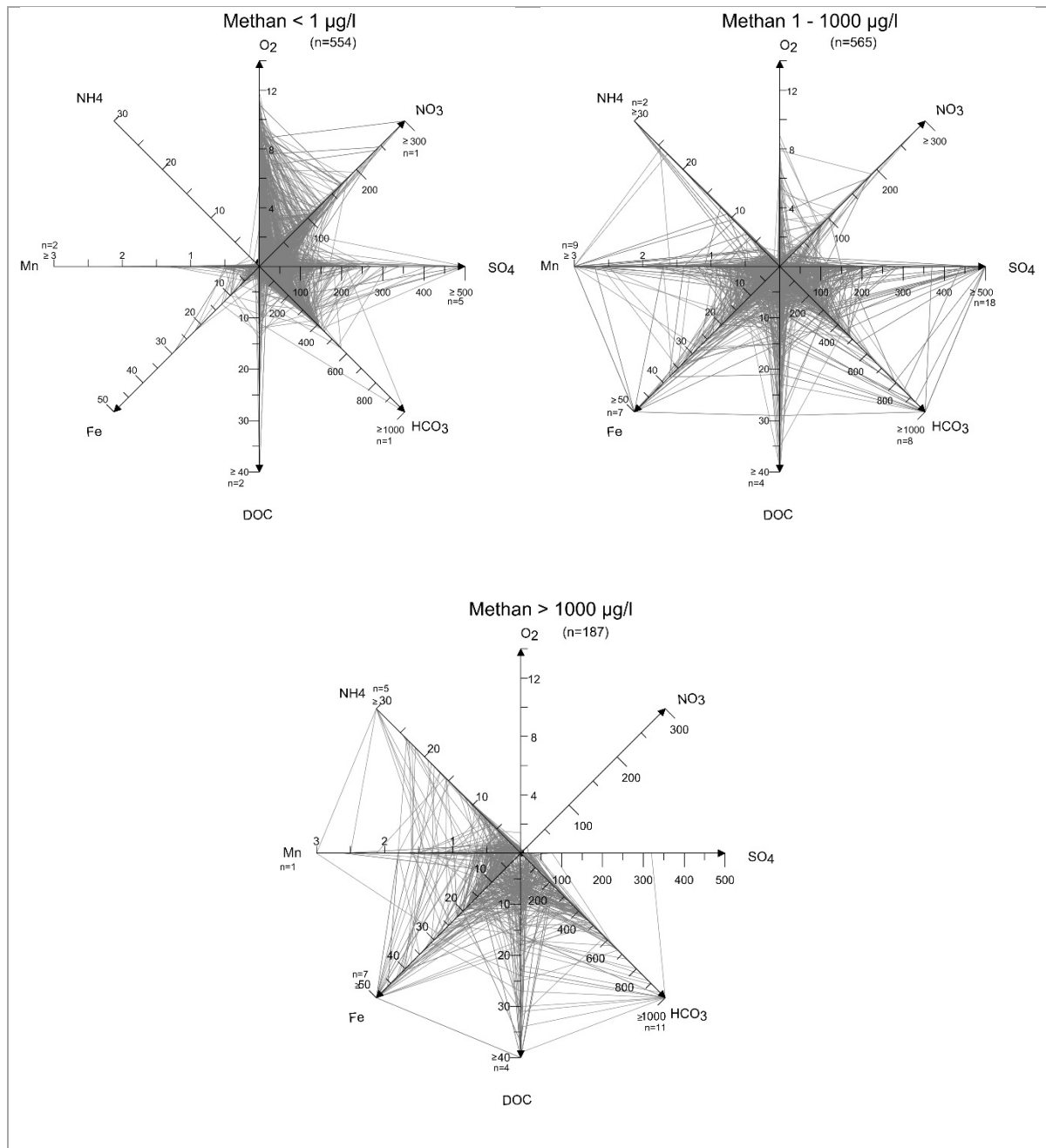
Abb. 15: Die Spider-Diagramme zeigen für sehr geringe, geringe bis mittlere und hohe Methangehalte die Konzentrationen an Sauerstoff (O 2 ), Nitrat (NO 3 ), Sulfat (SO 4 ), Hydrogenkarbonat (HCO 3 ), gelöstem organischen Kohlenstoff (DOC), Eisen (Fe), Mangan (Mn) und Ammonium (NH 4 ).
