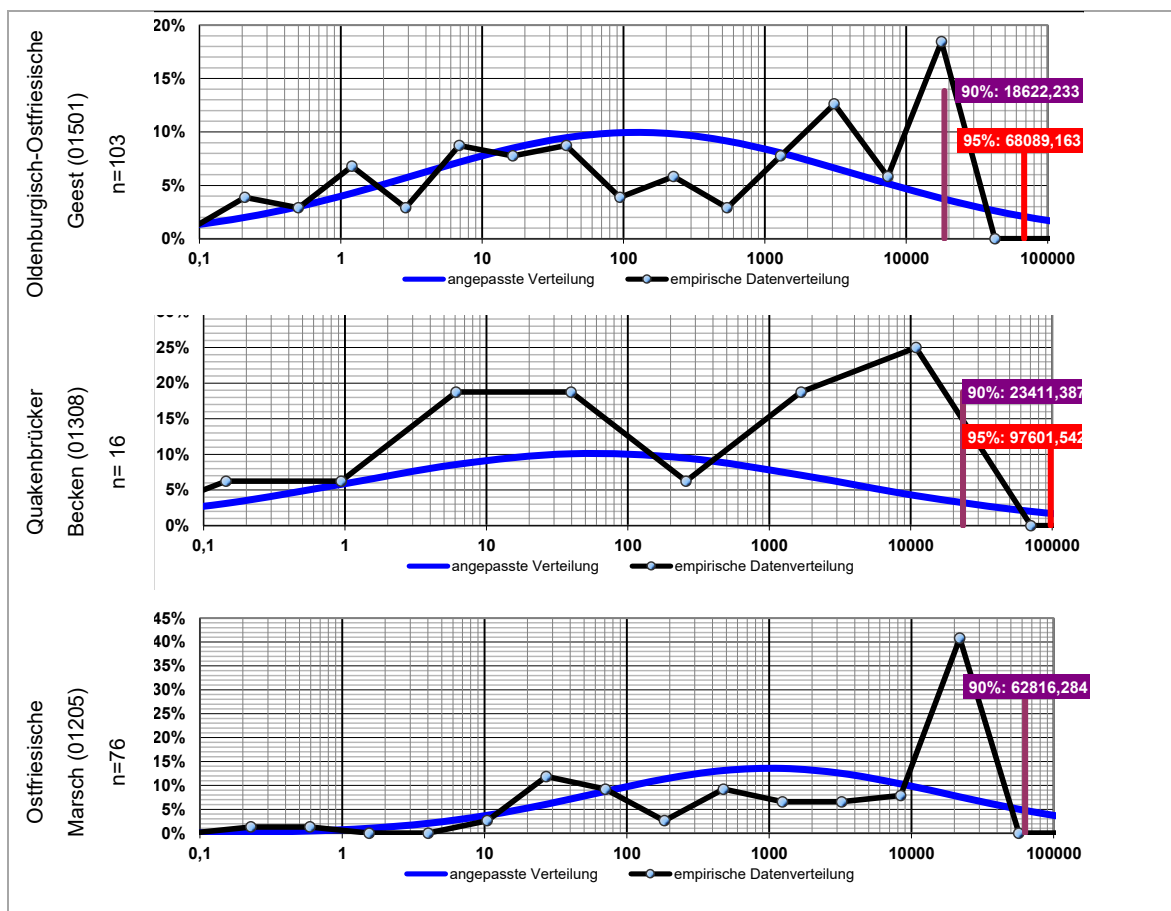
Abb. 17: Ableitung der Hintergrundwerte von Methan für drei Hydrogeologische Teilräume mit Hilfe des Wahrscheinlichkeitsnetzes (Excel-Makro Probnets). Die schwarze Linie zeigt das Histogramm der gemessenen Werte und die blaue Linie die angepasste Normalverteilung. In den lila bzw. roten Quadraten sind die berechneten 90%- bzw. 95%-Perzentile der angepassten Verteilung zu sehen.
