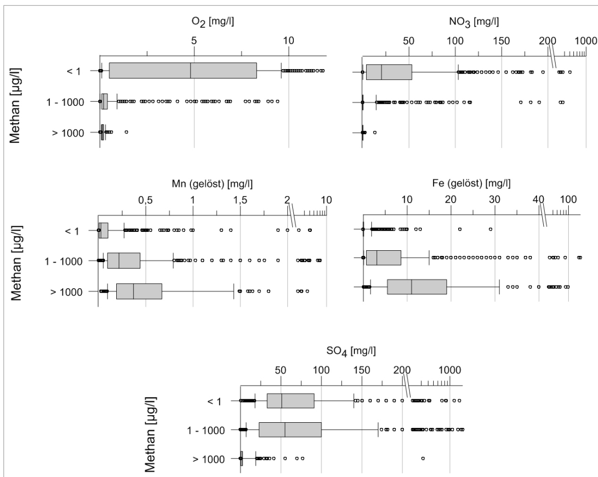
Abb. 12: Vergleich der Konzentrationen von Sauerstoff (O 2 ), Nitrat (NO 3 ), Mangan (gelöst), Eisen (gelöst) und Sulfat (SO 4 ) bei Proben mit sehr geringen ( <1 \mu\text{g/l} , n = 553 ), geringen bis mittleren (1–1000 \mu\text{g/l} , n = 565 ) und hohen Methankonzentrationen ( >1000 \mu\text{g/l} , n = 187 ).
