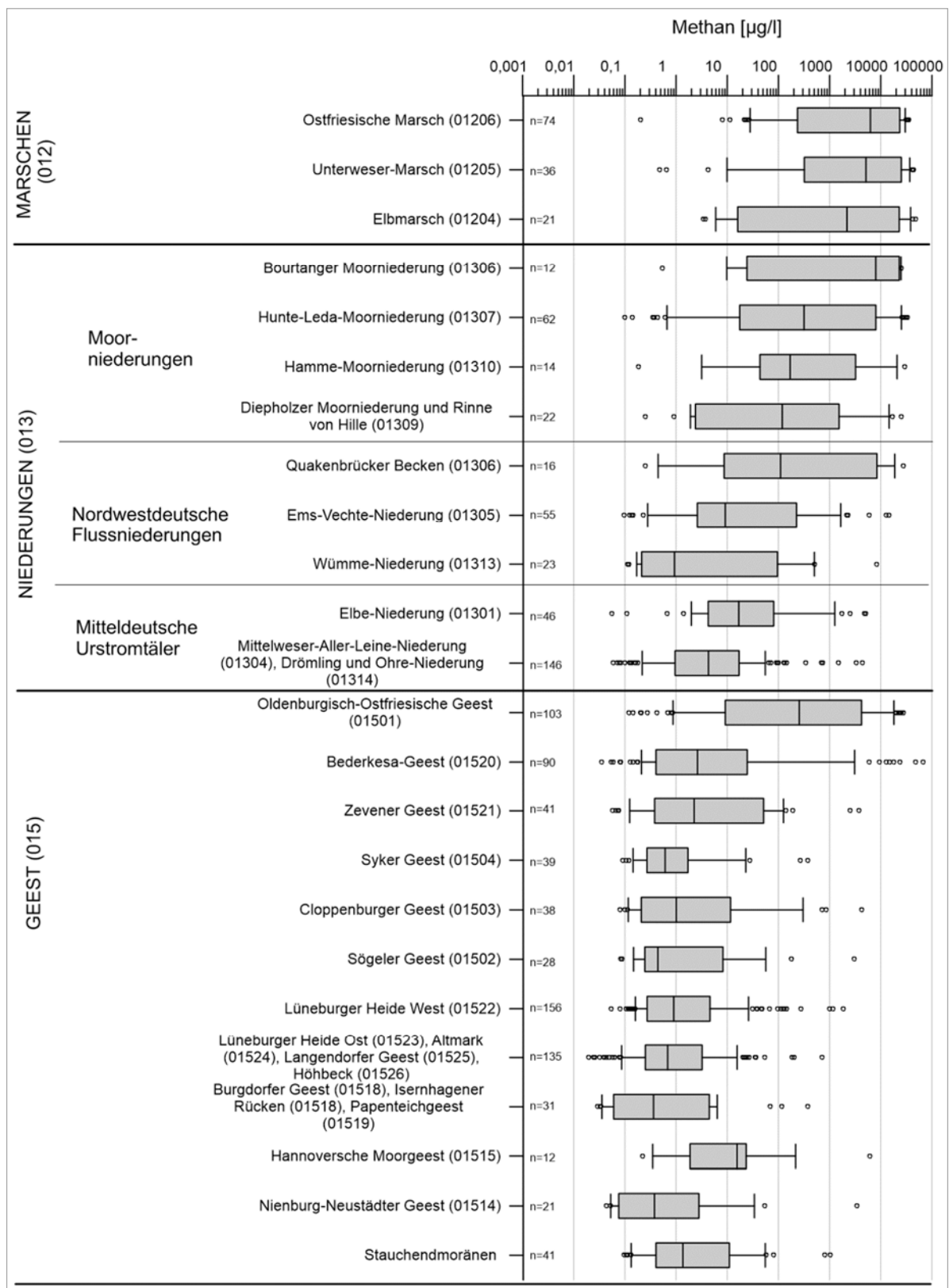
Abb. 20: Methan-Hintergrundwerte der Hydrogeologischen Teilräume des niedersächsischen Lockergesteinsgebietes (n = Anzahl der Messstellen). Die im südlichen Teil des Flachlandes liegenden Geestbereiche sind zu Stauchendmoränen aggregiert.
