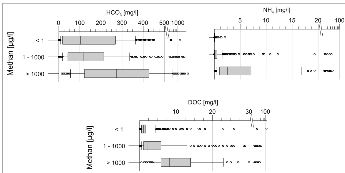
Abb. 14: Vergleich der Konzentrationen von Hydrogenkarbonat ( \text{HCO}_3^- ), Ammonium ( \text{NH}_4^+ ) und gelöstem organischen Kohlenstoff (DOC) für sehr geringe (<1 µg/l, n = 187), geringe bis mittlere (1–1000 µg/l, n = 553) und hohe Methankonzentrationen (>1000 µg/l, n = 565).
