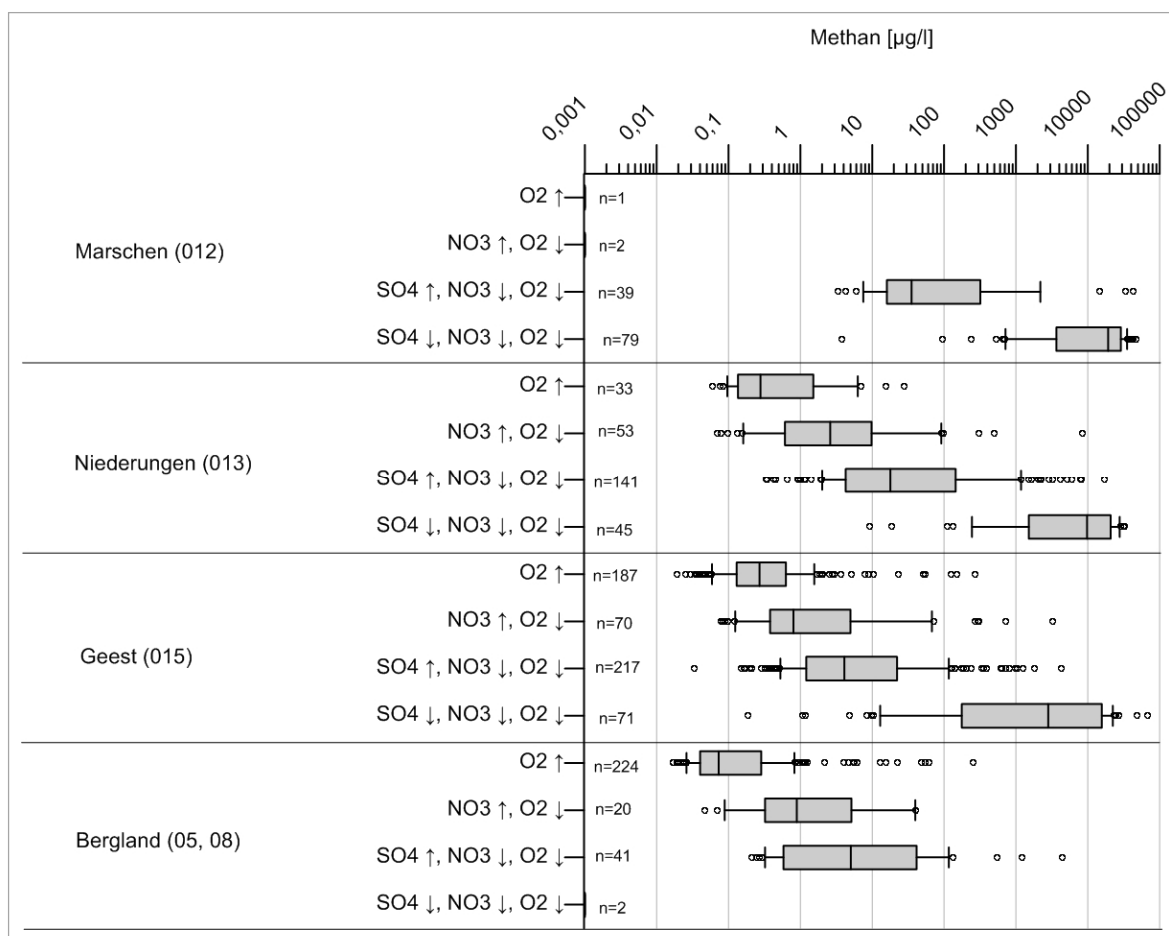
Abb. 19: Verteilung der Methankonzentrationen in den Hydrogeologischen Räumen Marschen, Niederungen und Geest sowie im niedersächsischen Bergland, untergliedert in die vier in Tabelle 5 definierten Reduktionsgrade.
