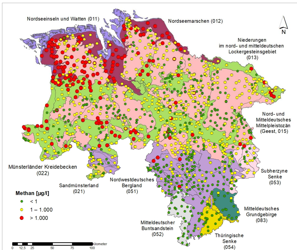
Abb. 16: Verteilung der Methankonzentrationen in den Hydrogeologischen Räumen Niedersachsens. Liegen Messstellen mit unterschiedlichen Filtertiefen nah aneinander, so liegt die niedrigere Konzentration grafisch über der höheren Konzentration, damit beide erkennbar sind. Diese Darstellung spiegelt somit nicht die Filtertiefe wieder.
