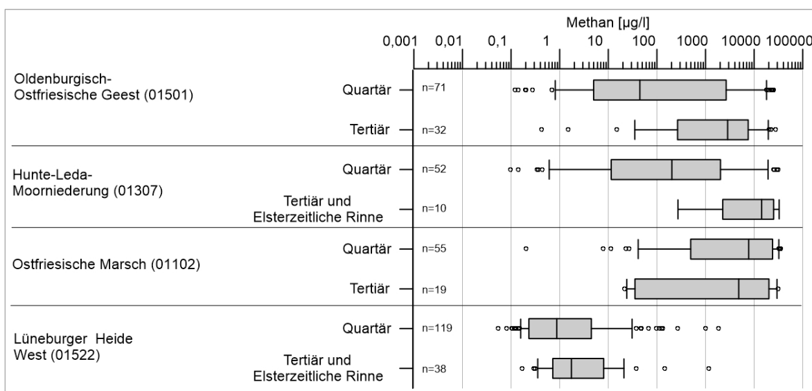
Abb. 21: Vergleich der Methankonzentrationen in den quartär- und tertiärzeitlichen Lockergesteins-Grundwasserleitern von vier Hydrogeologischen Teilräumen.
