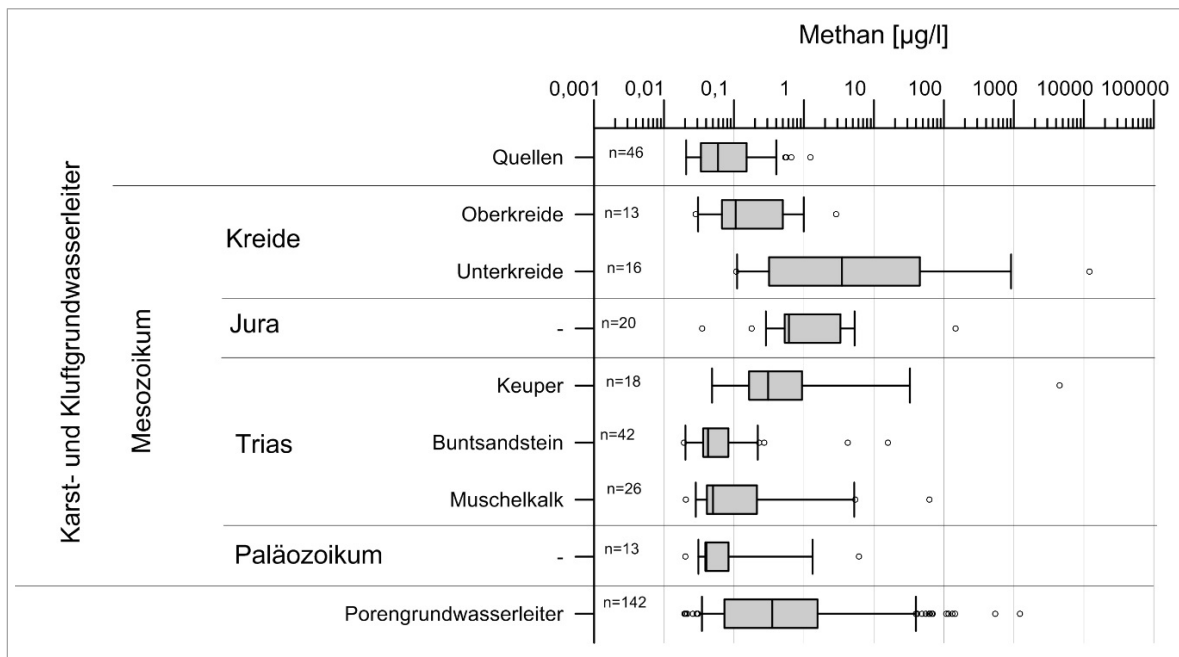
Abb. 22: Methankonzentrationen in den mesozoischen und paläozoischen Karst- und Kluftgrundwasserleitern (n = 148) sowie Porengrundwasserleitern (n = 142) des niedersächsischen Berglandes. Die Quellen werden gesondert gezeigt (n = 46).
