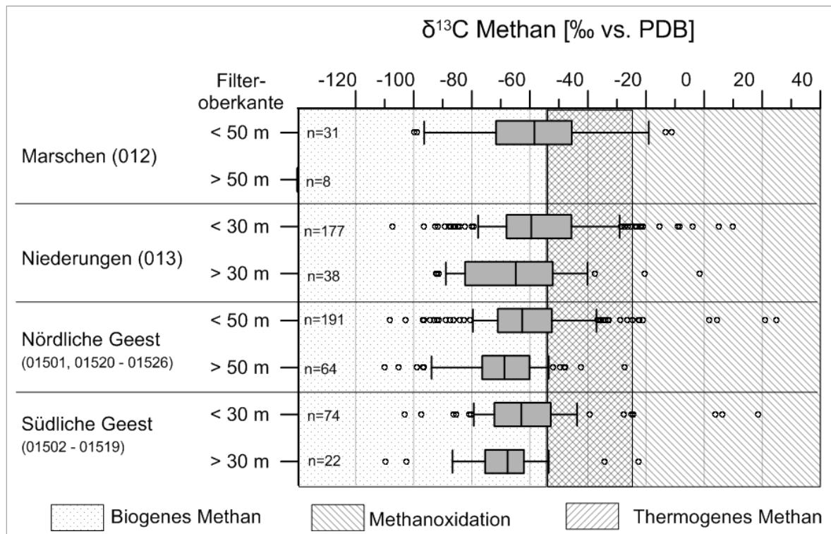
Abb. 24: Verteilung der \delta^{13}\text{C} -Werte von Methan in den flachen und tiefen Filtern in den Marschen, Niederungen und nördlichen bzw. südlichen Geestgebieten. Da die Schwankungsbreite bei Methankonzentrationen <1000 \mu\text{g/l} generell groß ist, werden nur diese Proben herangezogen.
