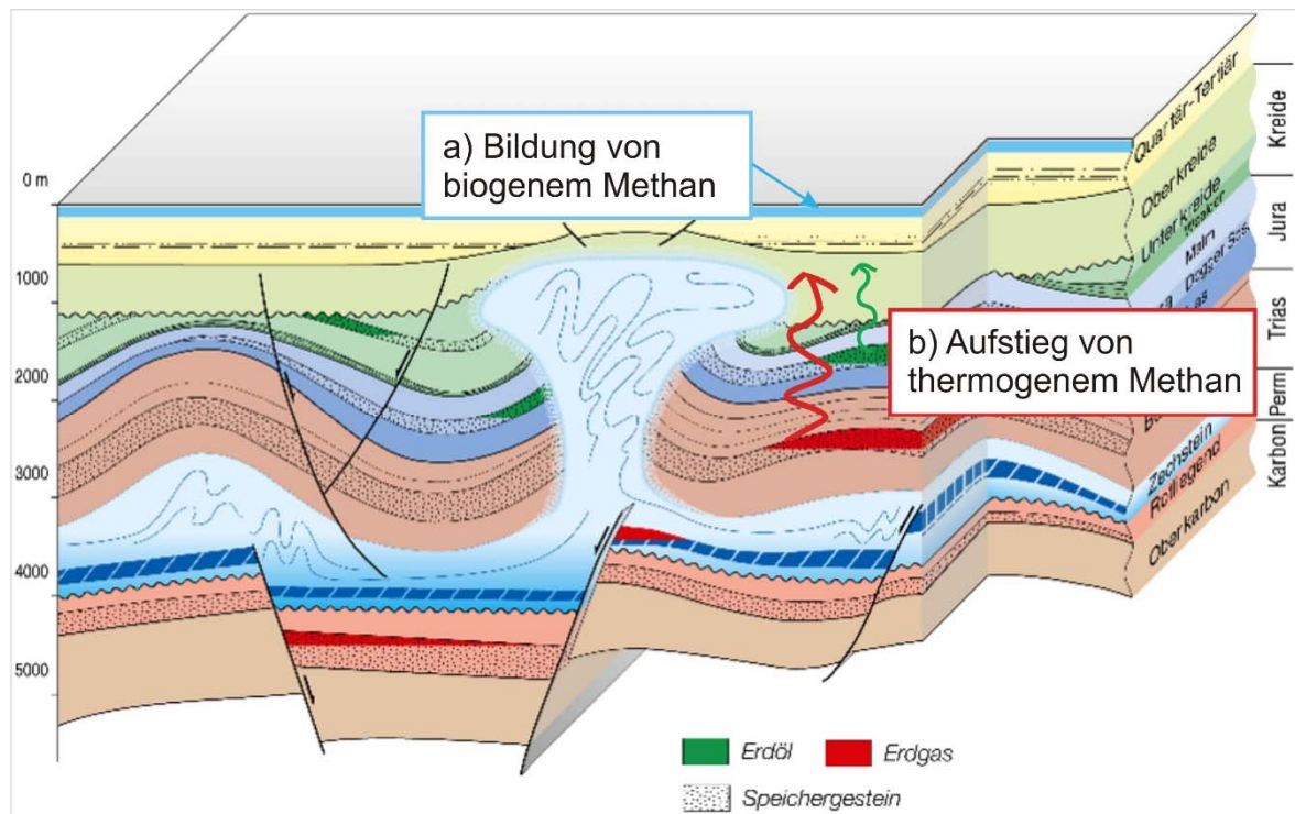
Abb. 1: Mögliche Eintragspfade von Methan ins Grundwasser (das oberflächennahe blaue Band): a) In-situ-Bildung im Grundwasser, b) Aufstieg von thermogenem Methan aus tieferliegenden Kohlenwasserstofflagerstätten.
